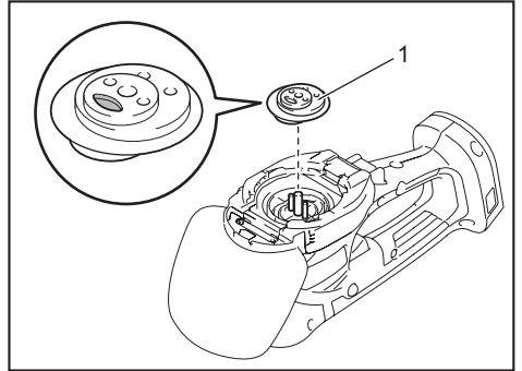
► 1. Crank
