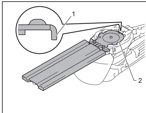
► 1. Griffes 2. Plaque-guide
