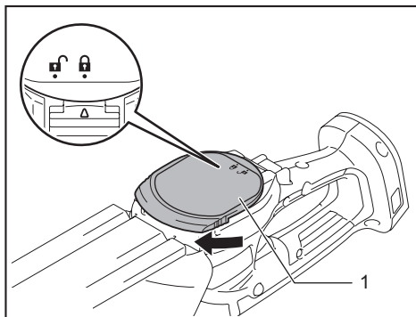
► 1. Undercover
